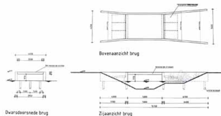
Dwarsdoorsnede brug
