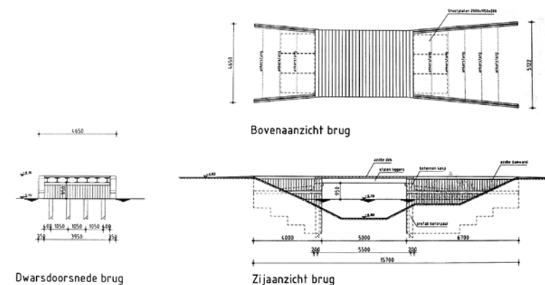
Dwarsdoorsnede brug
